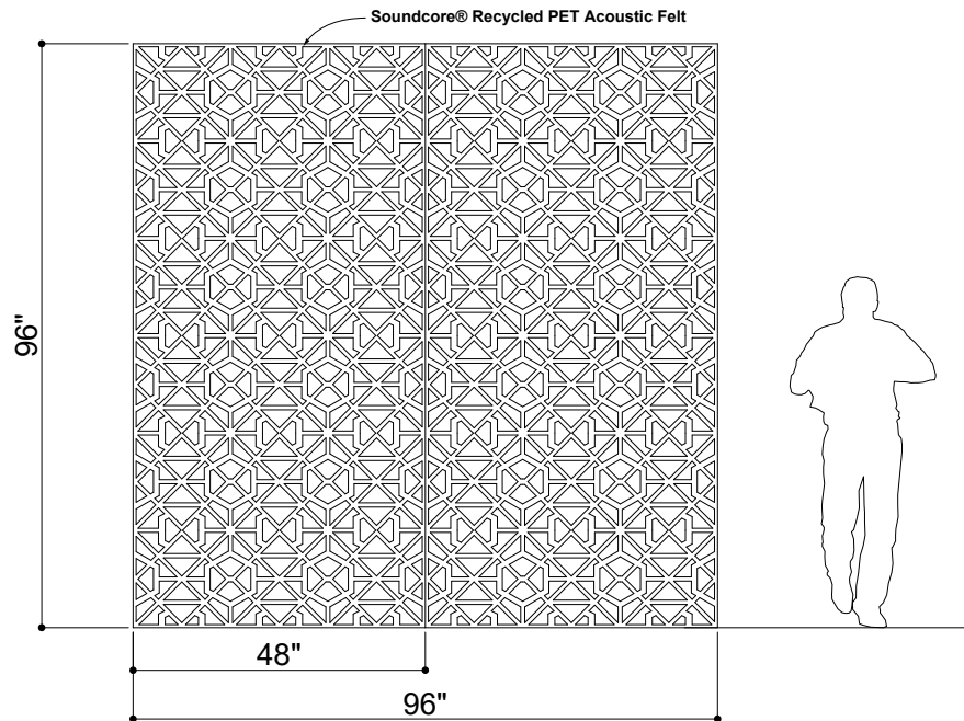
② ELEVATION 2
