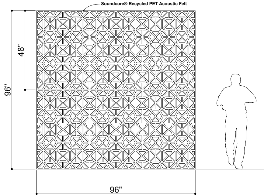
① ELEVATION 1
